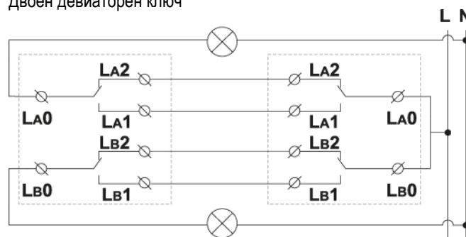
Схема на свързване Двоен девиаторен ключ
